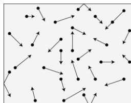
représentation microscopique d'un gaz
